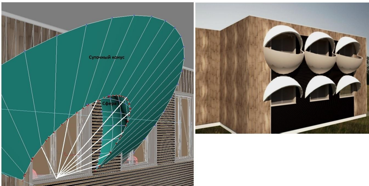
Рисунок 4 – Солнцезащитное устройство в виде сферы
