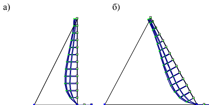
Рисунок 3 - Деформированные схемы подпорных стен а - с вертикальным расположением лицевой мембраны; б- с расположением лицевой мембраны под углом наклона \varphi = 28^\circ
