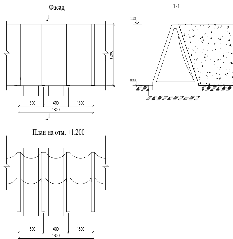
Рисунок 1 - Конструктивное решение подпорной стенки
