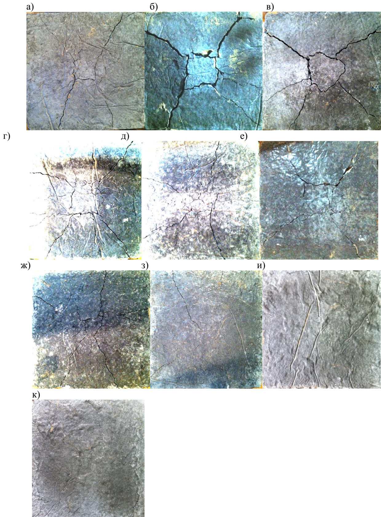
Рисунок 1 – Подошвы моделей фундаментов после испытания: (а) – Ф-1-5, (б) – Ф-2-5, (в) – Ф-3-5, (г) – Ф-4-5, (д) – Ф-5-7, (е) – Ф-6-7, (ж) – Ф-7-7, (з) – Ф-8-7, (и) – Ф-9-10, (к) – Ф-10-10
