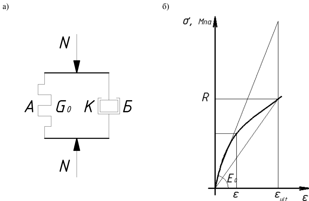
Рисунок 1 – Схема реологической модели Кельвина-Фойгта (а) и общая физическая модель деформирования древесины (б)
