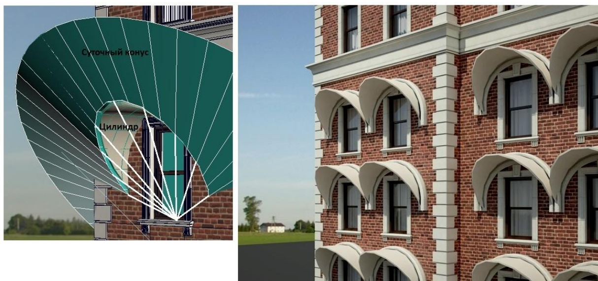
Рисунок 5 – Солнцезащитное устройство в виде цилиндра
