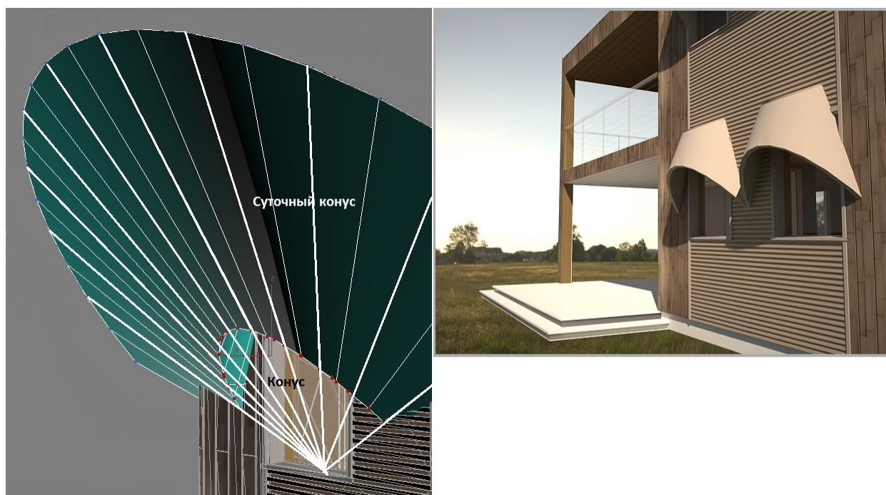
Рисунок 6 – Солнцезащитное устройство в виде конуса
