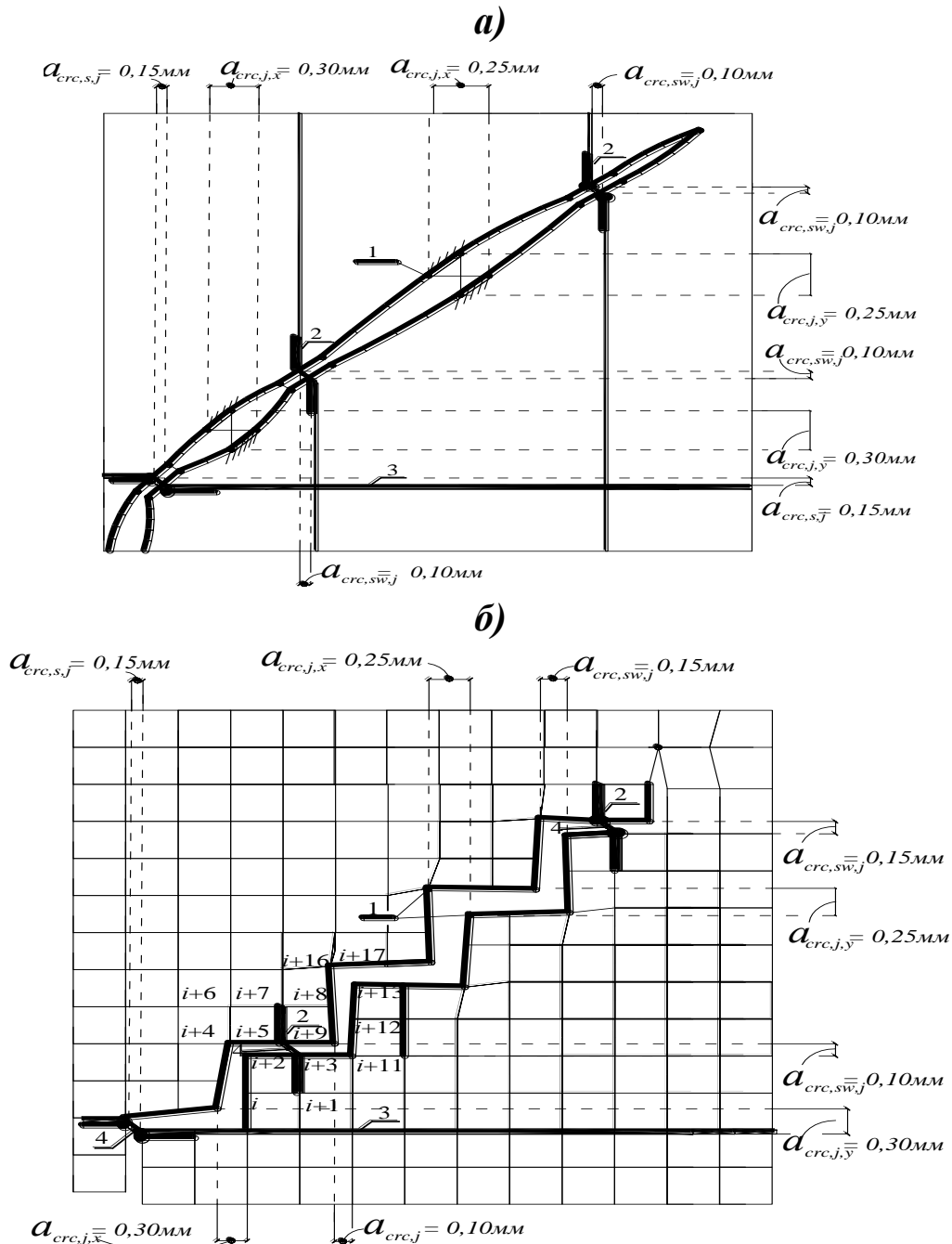
Рисунок 3 – Предлагаемая модель трещины: а) – действительная трещина; б) – моделируемая с помощью расшивки КЭ и деформационного воздействия \Delta = a_{cr,j}
