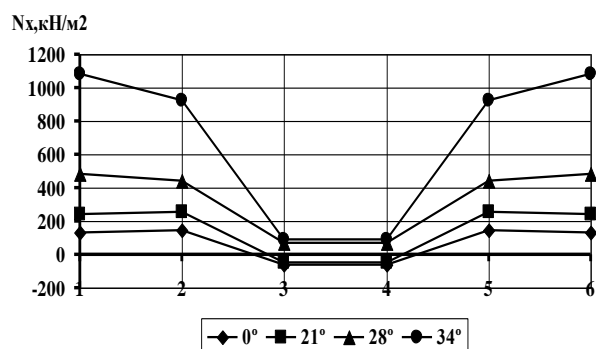
Рисунок 5 - Горизонтальные нормальные напряжения в лицевой мембране при различных углах наклона а - в сечении на высоте 0.05м от основания; б - в сечении на высоте 0.45м от основания; в - в сечении на высоте 0.85м от основания; г - в сечении на высоте 1.150м от основания
