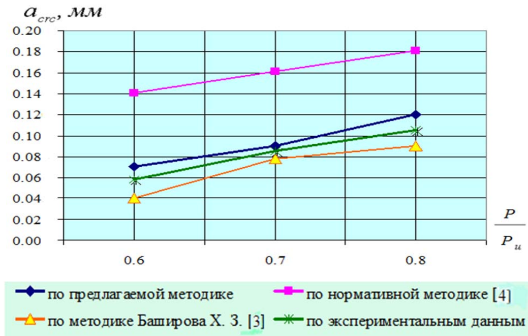
Рисунок 4 – Графики зависимости « a_{crc} - P/P_u » для конструкции второй серии БС-II-2,7-100-06
