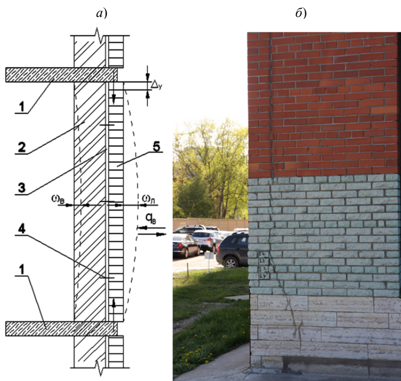
Рисунок 1 – Схема работы зацементированного между дисками перекрытий лицевого каменного слоя (а) и его выпучивание из плоскости при внецентренном загрузении (б): 1 – диски перекрытий; 2 – внутренний каменный слой; 3 – воздушный зазор; 4 – гибкие анкера; 5 – каменный лицевой слой
