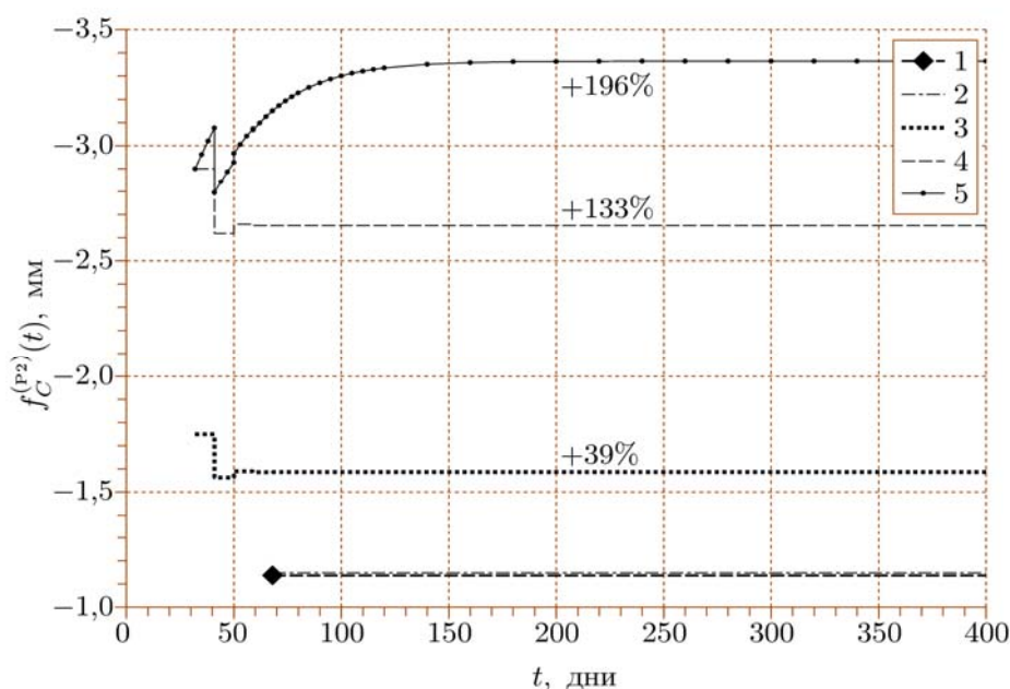
Рисунок 2 – Стрела прогиба ригеля второго этажа (от нагрузок на этапе возведения): 1 – по МКЭ; 2 – по МСАЭ; 3 – с учётом последовательности возведения; 4 – с учётом твердения бетона; 5 – с учётом ползучести бетона
