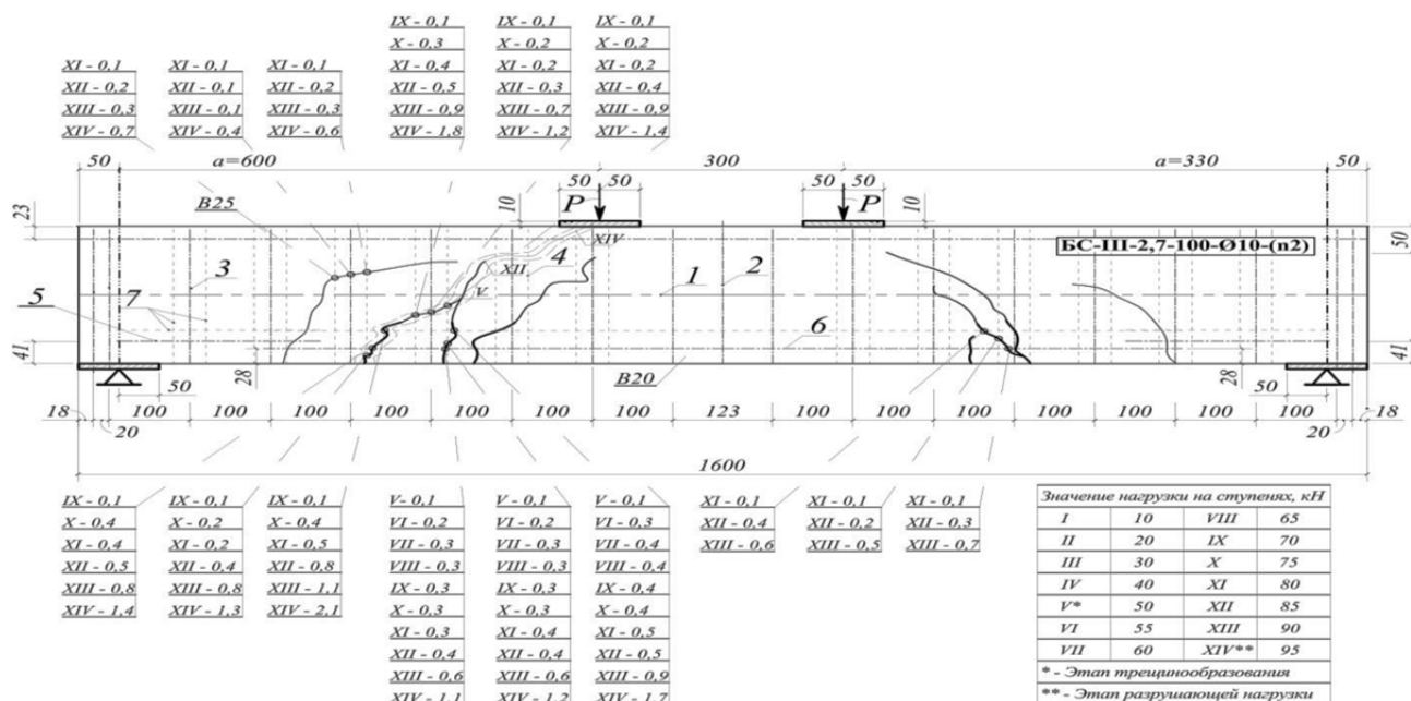
Рисунок 1 – Схема образования и раскрытия трещин в опытной конструкции третьей серии БС-III-2,7-100-Ø10-(n2): 1 – средняя нейтральная ось; 2 – вертикальная ось симметрии образца; 3 – поперечные хомуты диаметром 6 мм из стали А240С; 4 – поперечные хомуты диаметром 10 мм из стали А240С; 5 – геометрические оси нижней рабочей арматуры в приопорной зоне 2Ø10А400С; 6 – геометрические оси нижней рабочей арматуры в середине балки 2Ø16А400С; 7 – дополнительные оси для замера трещин, смещенные от осей арматуры на расстояние двух диаметров
