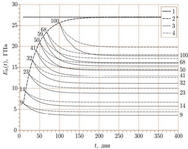
Рисунок 1 – Модуль упругости бетона E_b : 1 – начальный модуль; 2 – с учётом твердения: E_b(t) = E_0 \cdot (1 - e^{-\alpha t}) ; 3 – при изгибе с учётом ползучести: E_{b1}(t_1; t) = E_{b0}(t_1) \cdot B_1(t_1; t) ; 4 – при растяжении-сжатии с учётом ползучести: E_{b2}(t_1; t) = E_{b0}(t_1) \cdot B_2(t_1; t)
