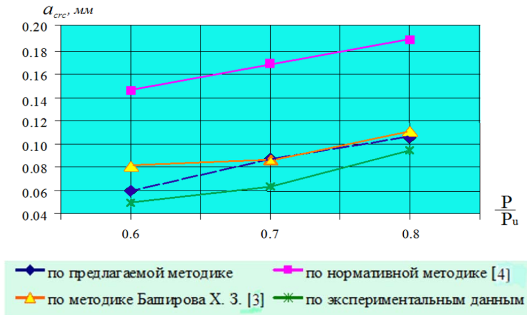
Рисунок 3 – Графики зависимости « a_{crc} - P/P_u » для конструкции пятой серии БС-V-2-100-06
