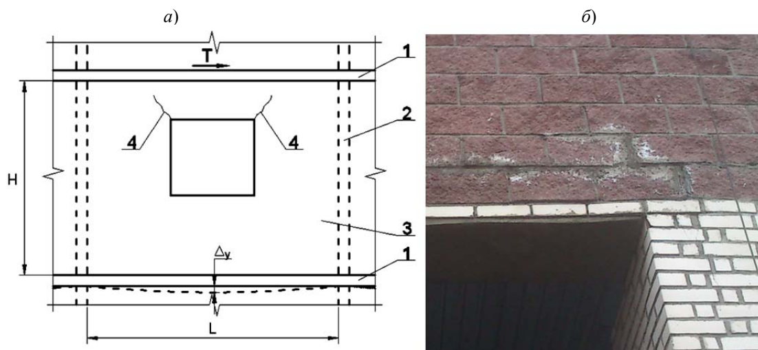
Рисунок 2 – Схема работы облицовочного слоя в его плоскости (а) с образованием косых трещин (б): 1 – диски перекрытий; 2 – внутренние поперечные стены; 3 – облицовочный кирпичный слой с оконными проёмами; 4 – трещины
