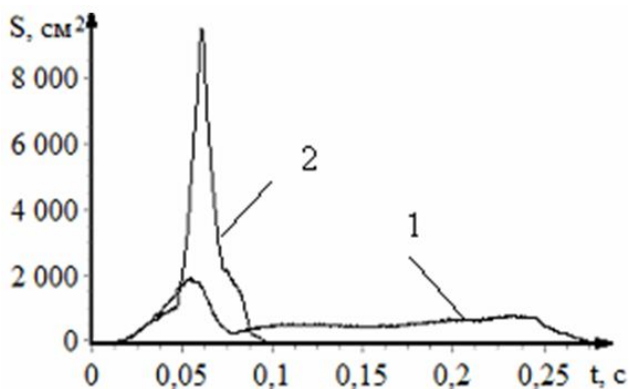
Рисунок 4 – Динамика площади фронта горения в полном цилиндре (1) и при диафрагме (2)
