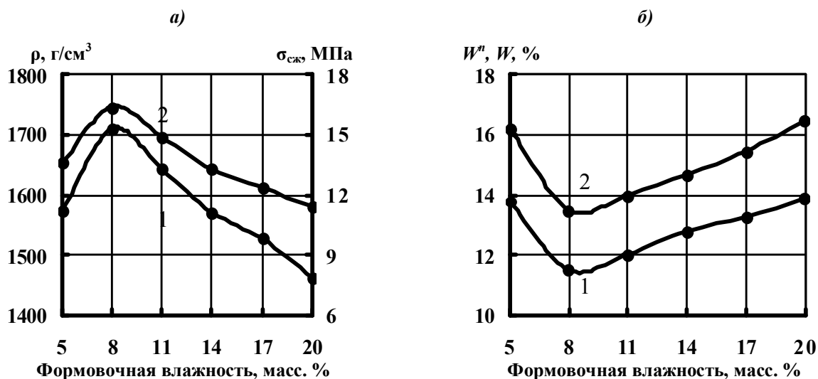
Рисунок 1 – Зависимость физико-механических свойств строительной керамики от формовочной влажности сырца на основе кислой глины:
