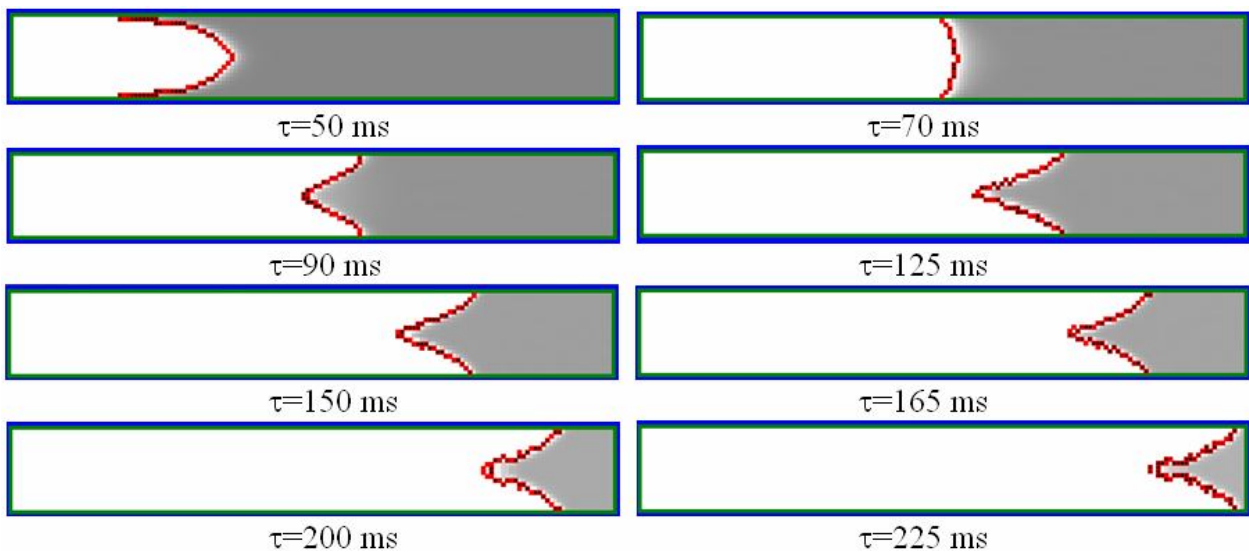
Рисунок 3 – Динамика взрыва в полом цилиндре
