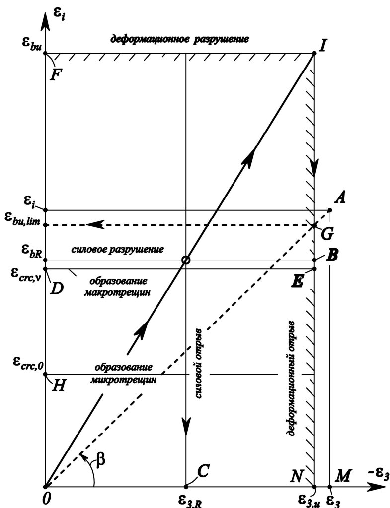
Рисунок 5 – Диаграмма механического состояния для оценки возможного вида разрушения бетона
