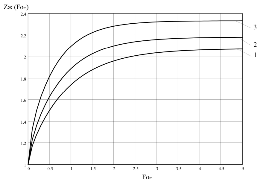
Рисунок 3 – Концентрация переносимого компонента в жидкой фазе F_{0m} от 0 до 10; K_m=0,1 ; Bi_m=0,5; 1; 1,5; 2; 3
