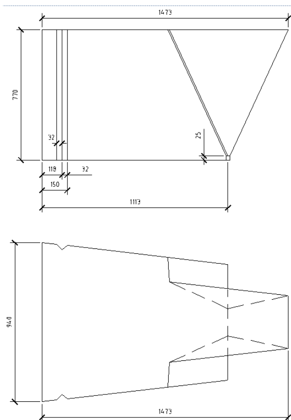
Рисунок 5 – Конструкция блока №2
