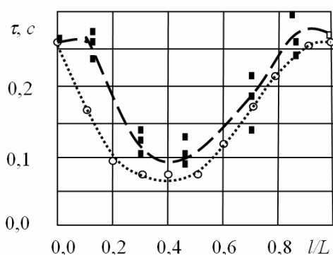
Рисунок 7 – Длительность времени выгорания в зависимости от положения диафрагмы с диаметром 65 мм
