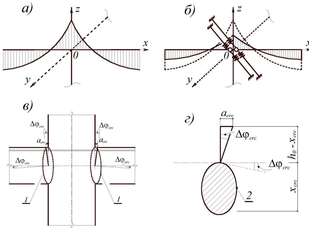
Рисунок 3 – К учету повышенной деформативности узлового сопряжения рамного железобетонного узла при его проектировании (эпюры моментов вдоль оси u условно не показаны): а – расчетная схема с жестким сопряжением, принятая в строительной механике; б – то же, при учете податливости сопряжения; в – возникновение трещин в углах узла, вызванное концентрацией напряжений и приводящее к повышенной деформативности узлового сопряжения; з – определение дополнительного угла поворота \Delta\varphi_{crc} . 1 – зоны повышенной деформативности; 2 – зоны кинематического поворота в сжатом бетоне
