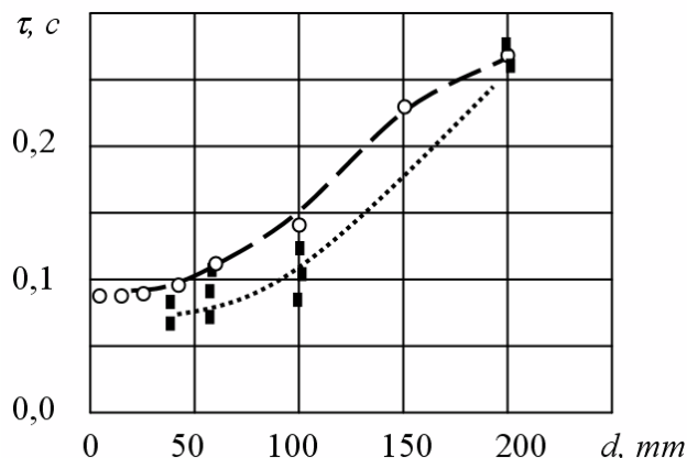
Рисунок 5 – Зависимость времени выгорания от диаметра отверстия на диафрагме:
