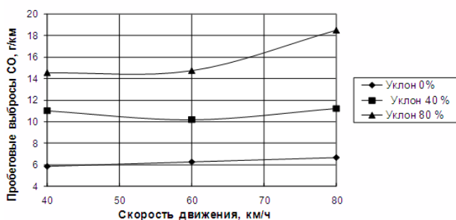
Рисунок 1 – Зависимость выбросов окиси углерода грузовым автомобилем массой до 3,5 – 12 т с дизельным двигателем от величины продольного уклона
