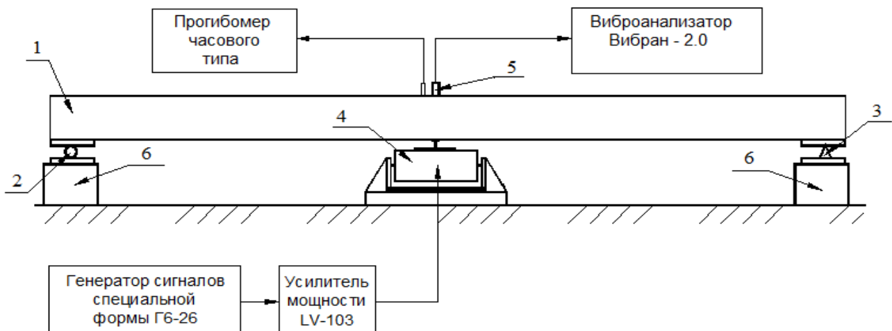
Рисунок 1 – Функциональная схема испытательного стенда: 1 – контролируемая балка; 2, 3 – подвижная и неподвижная шарнирные опоры; 4 – ударное устройство – возбудитель собственных поперечных колебаний; 5 – виброанализатор спектра колебаний «Вибран-2»; 6 – силовые опоры
